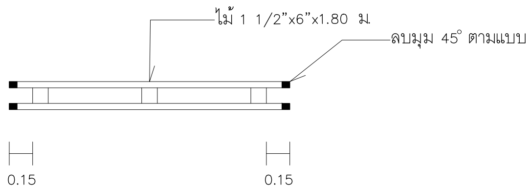
แปลนแสดงรูปตัดด้านข้างตามยาว
