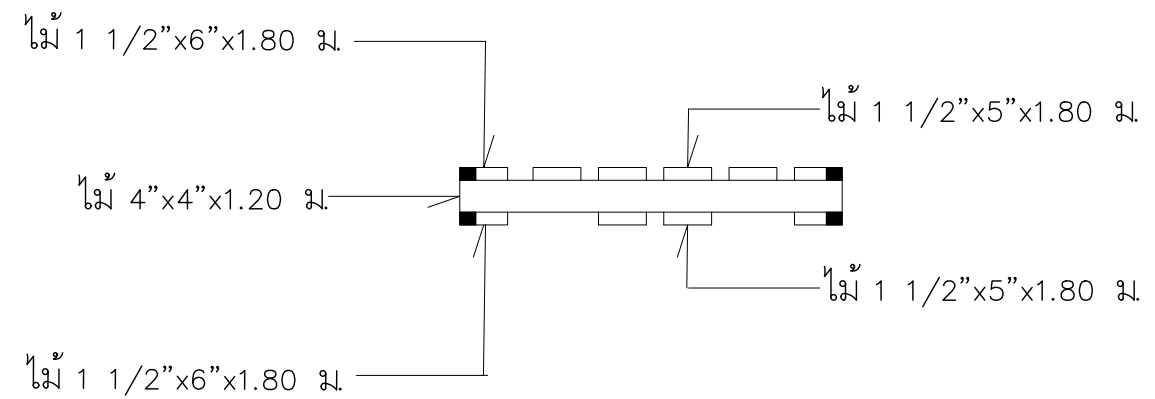
แปลนแสดงรูปตัดด้านข้างตามกว้าง
